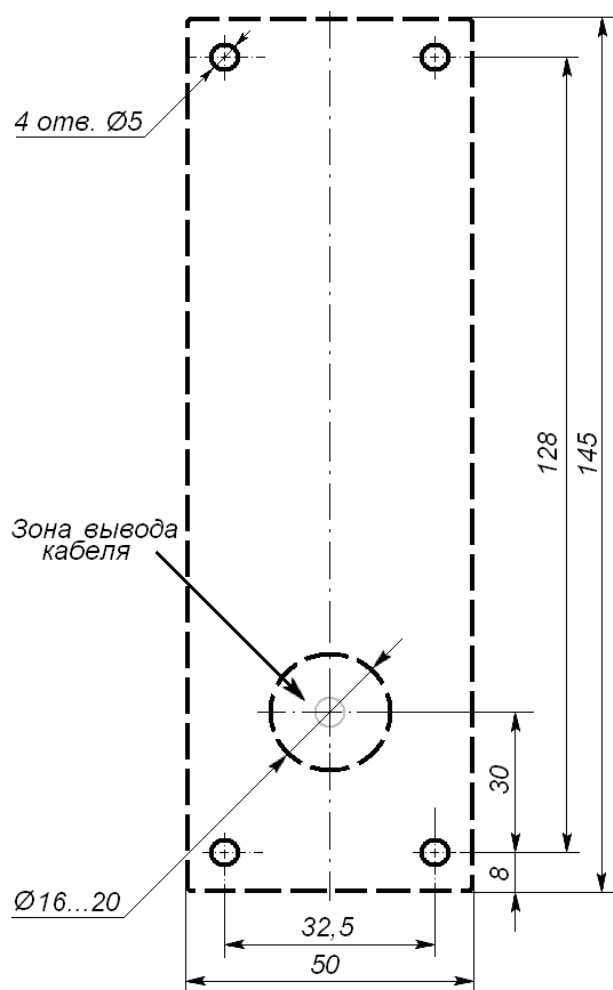
Рисунок 3 Разметка отверстий для установки контроллера (штрих-пунктиром показаны габариты корпуса контроллера)
