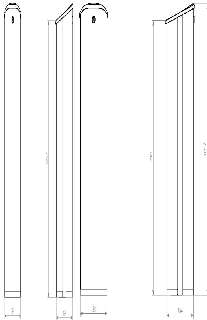
Рисунок 3 – Габаритные размеры картоприёмника
