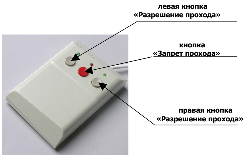
Рисунок 3 – Пульт управления
