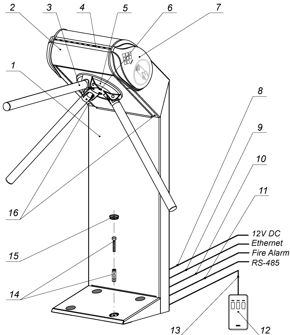
Рисунок 2. Устройство ЭП:
