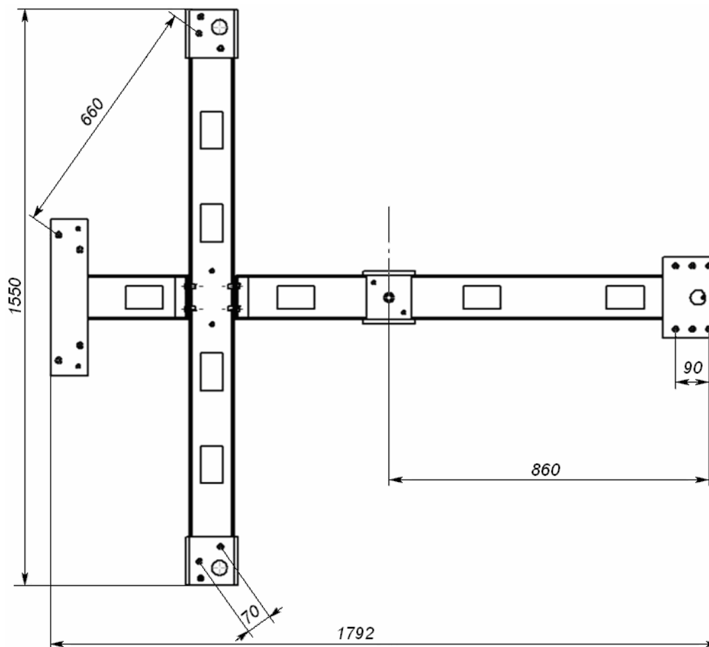
Рисунок 1. Габаритные и установочные размеры рамы
