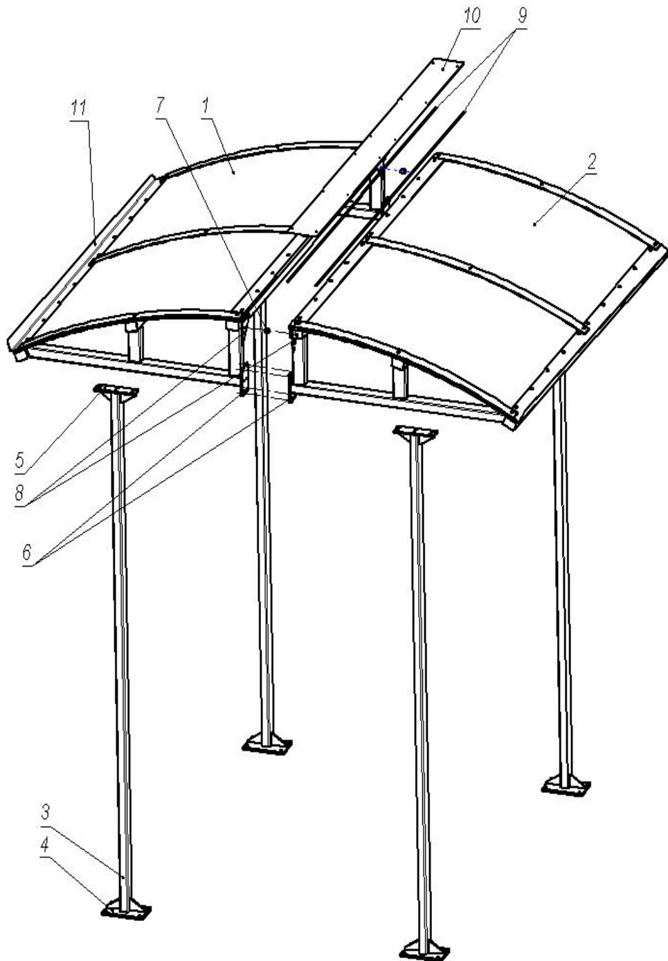
Рисунок 1 – Устройство крыши:
