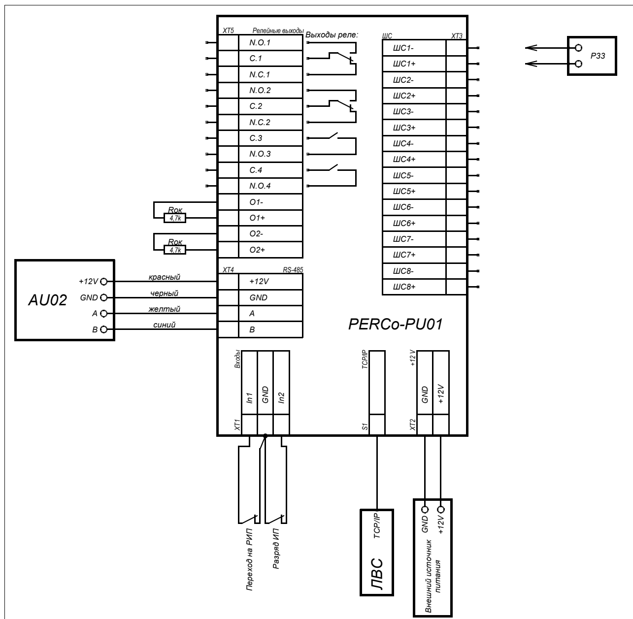
Рисунок Е.1 – Схема подключения ППКОП PERCo-PU01 при проверке технического состояния
