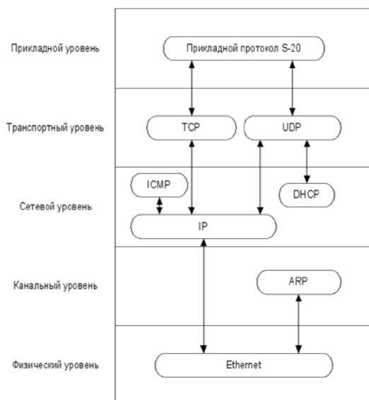
Рис. 2. Стек протоколов, используемых для обмена в системе
