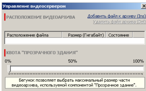
Рис. 6. Управление видеосервером
