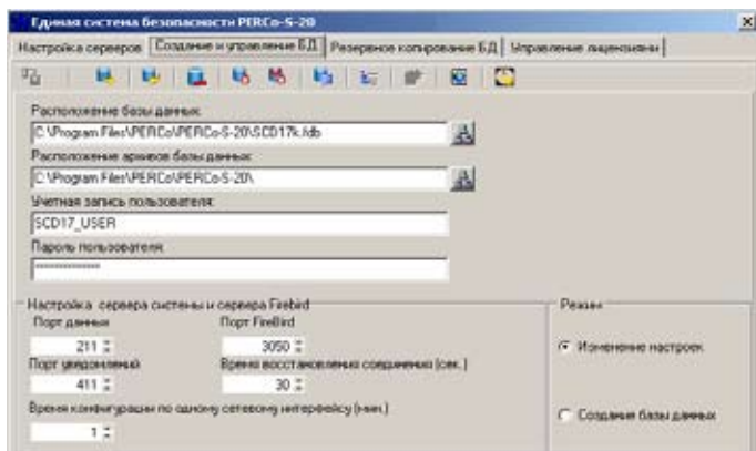
Рис. 6.
