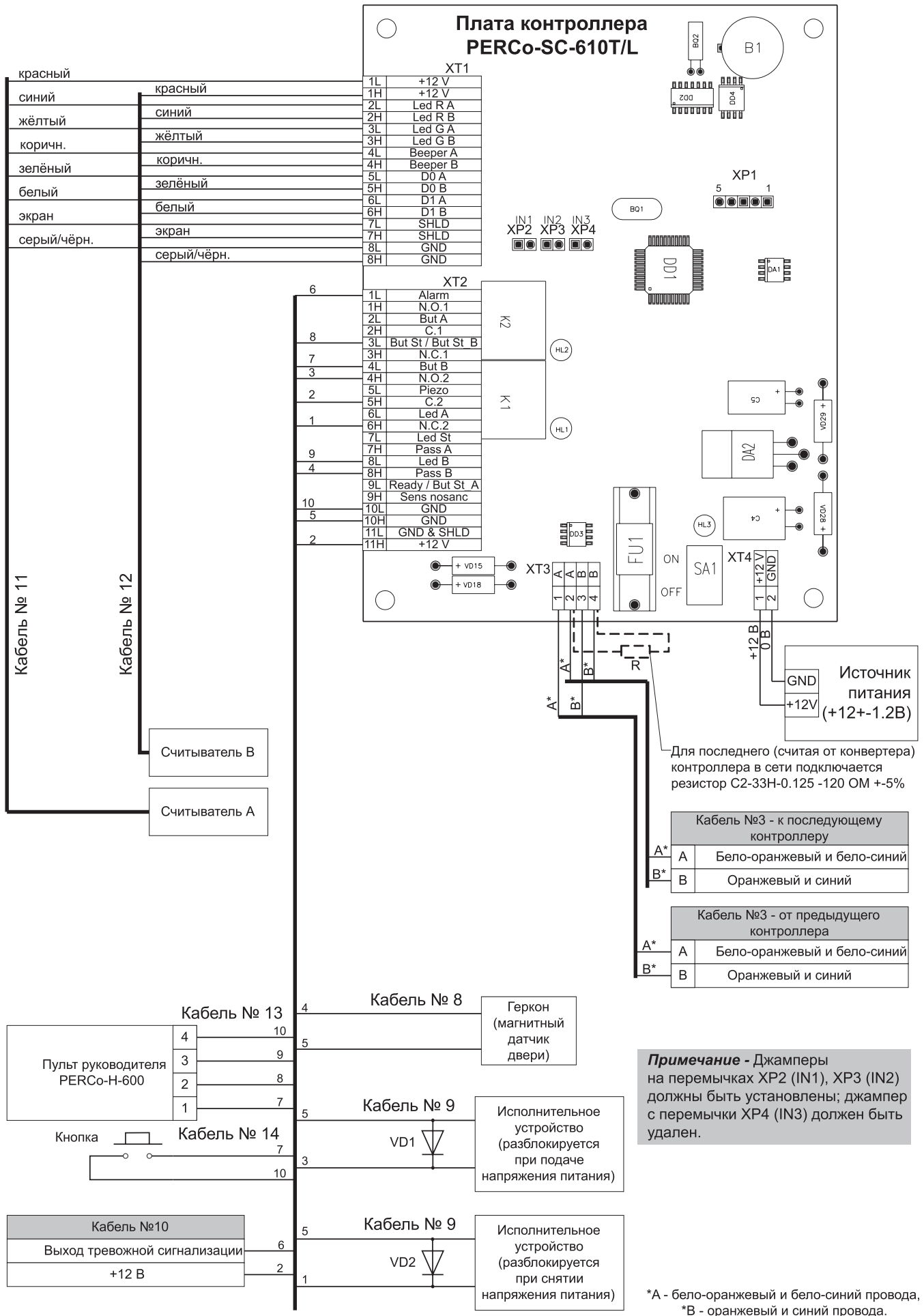
Схема 15- Схема монтажа контроллера PERCo-SC-610T/L (вариант "Замок" — оба считывателя привязаны к исполнительному устройству "B").
