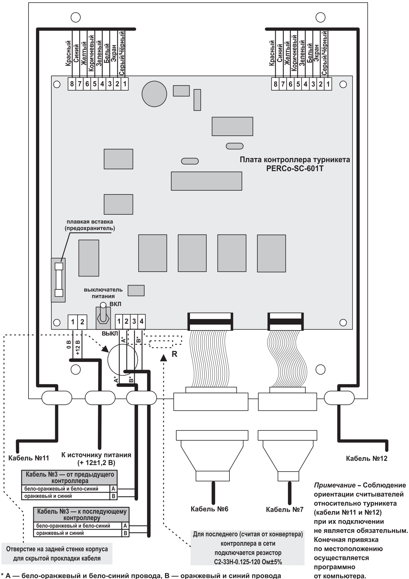
Схема 8- Схема монтажа контроллера турникета PERCo-SC-601T
