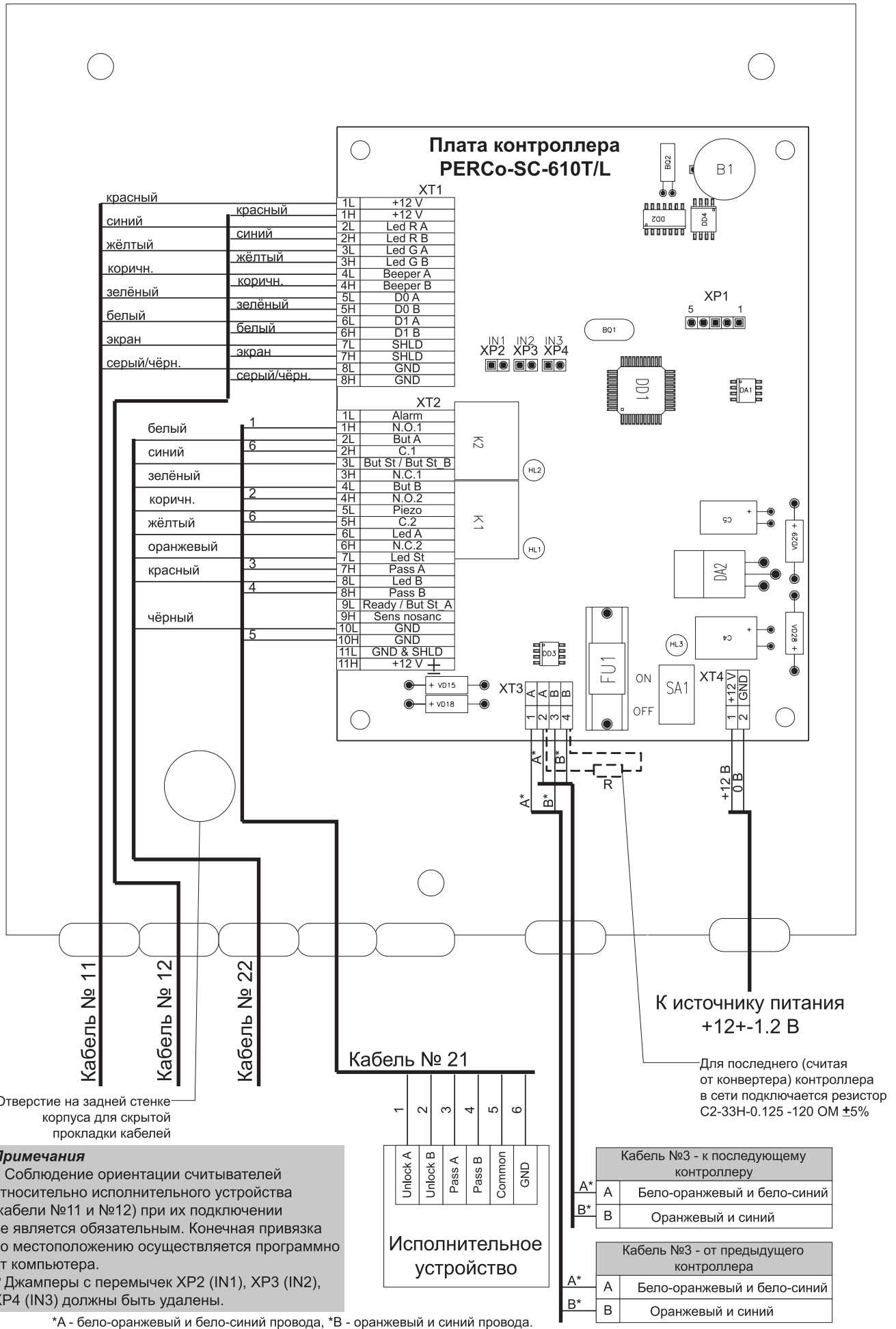
Схема 13- Схема монтажа контроллера PERCo-SC-610T/L (вариант "Турникет")
