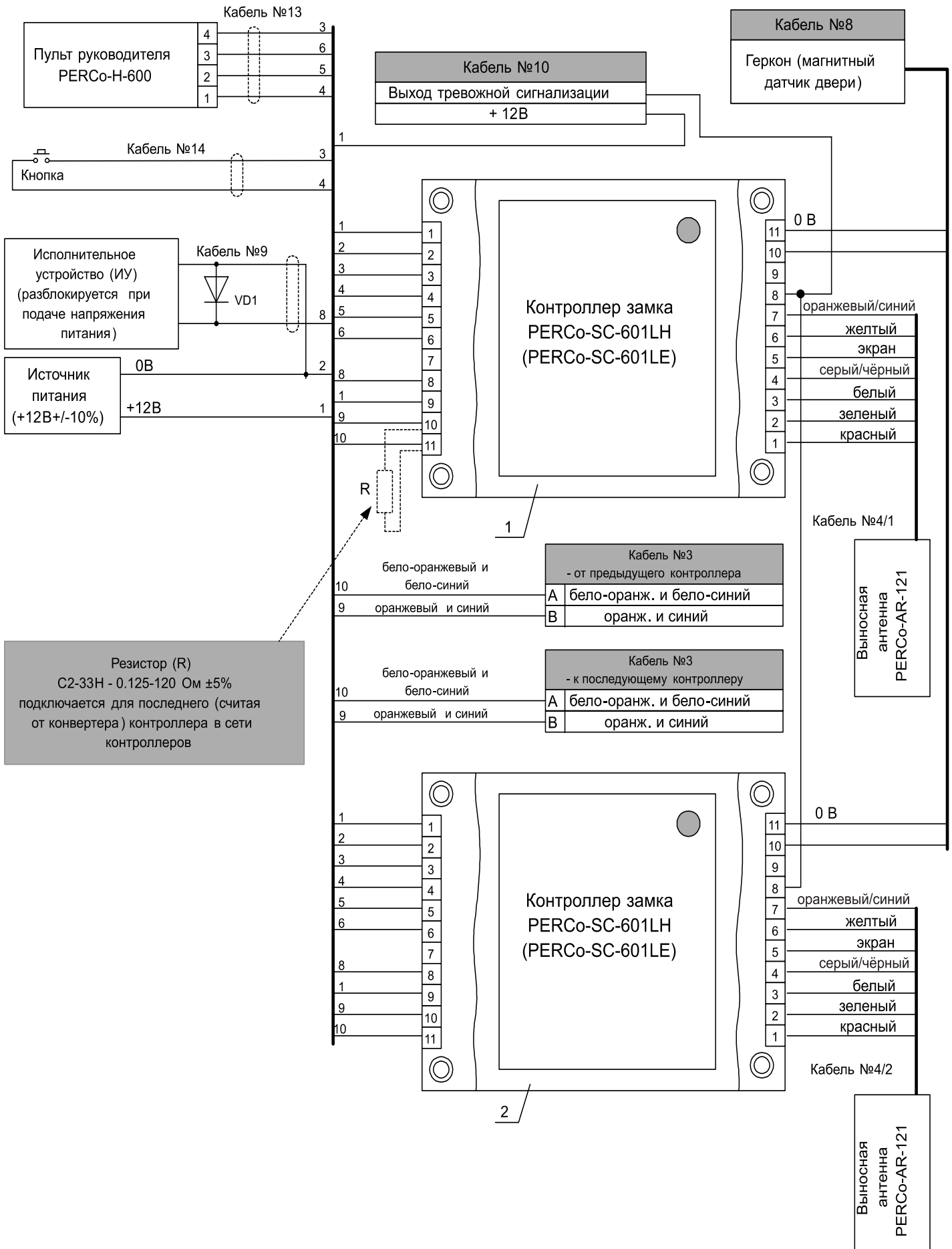
Схема 4в- Схема монтажа контроллеров замка PERCo-SC-601LH (LE) при организации входа и выхода в помещение по бесконтактным картам доступа
