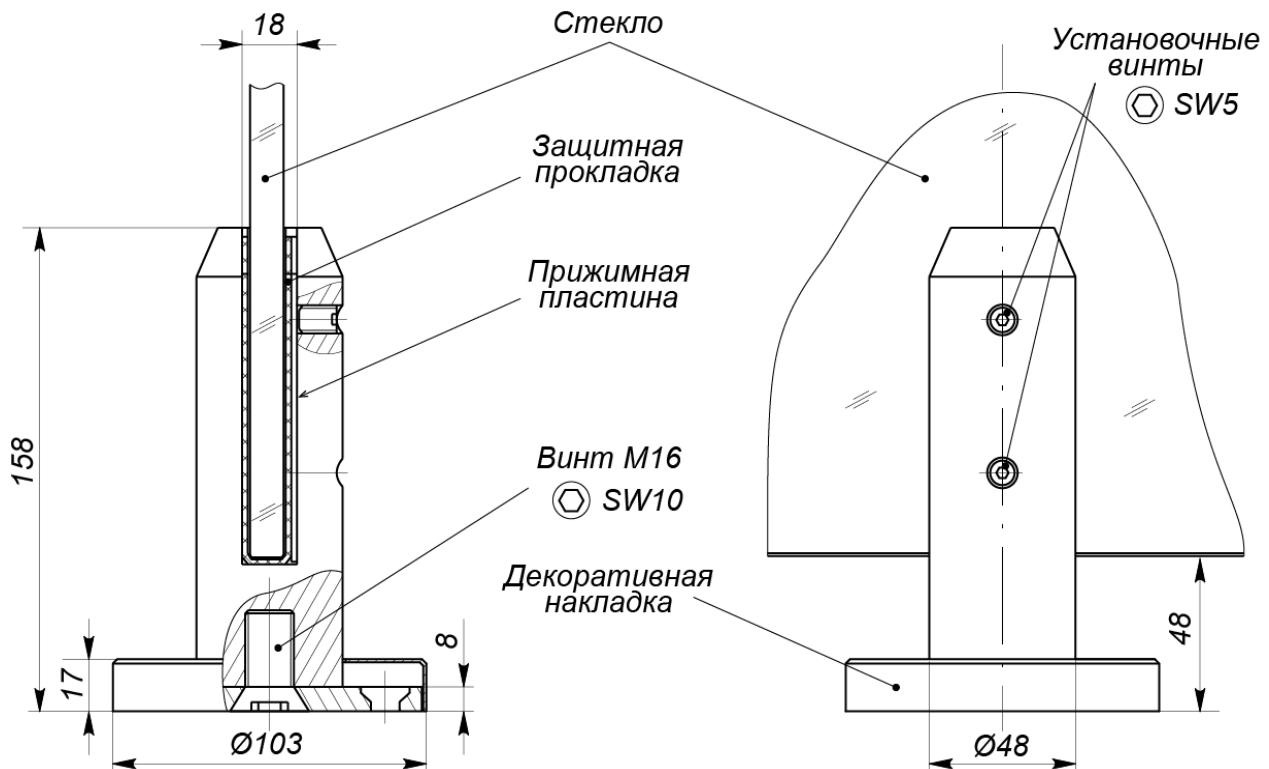
Рисунок 1. Внешний вид и размеры мини-стойки PERCo-BH06 2-00
