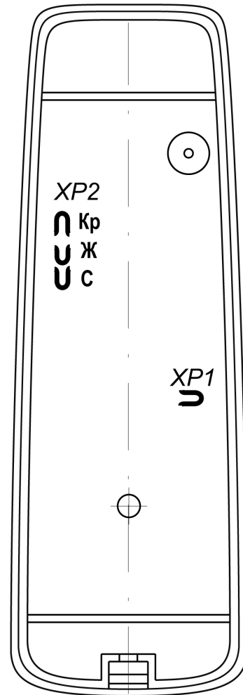
Рисунок 3. Расположение перемычек на тыльной стороне контроллера
