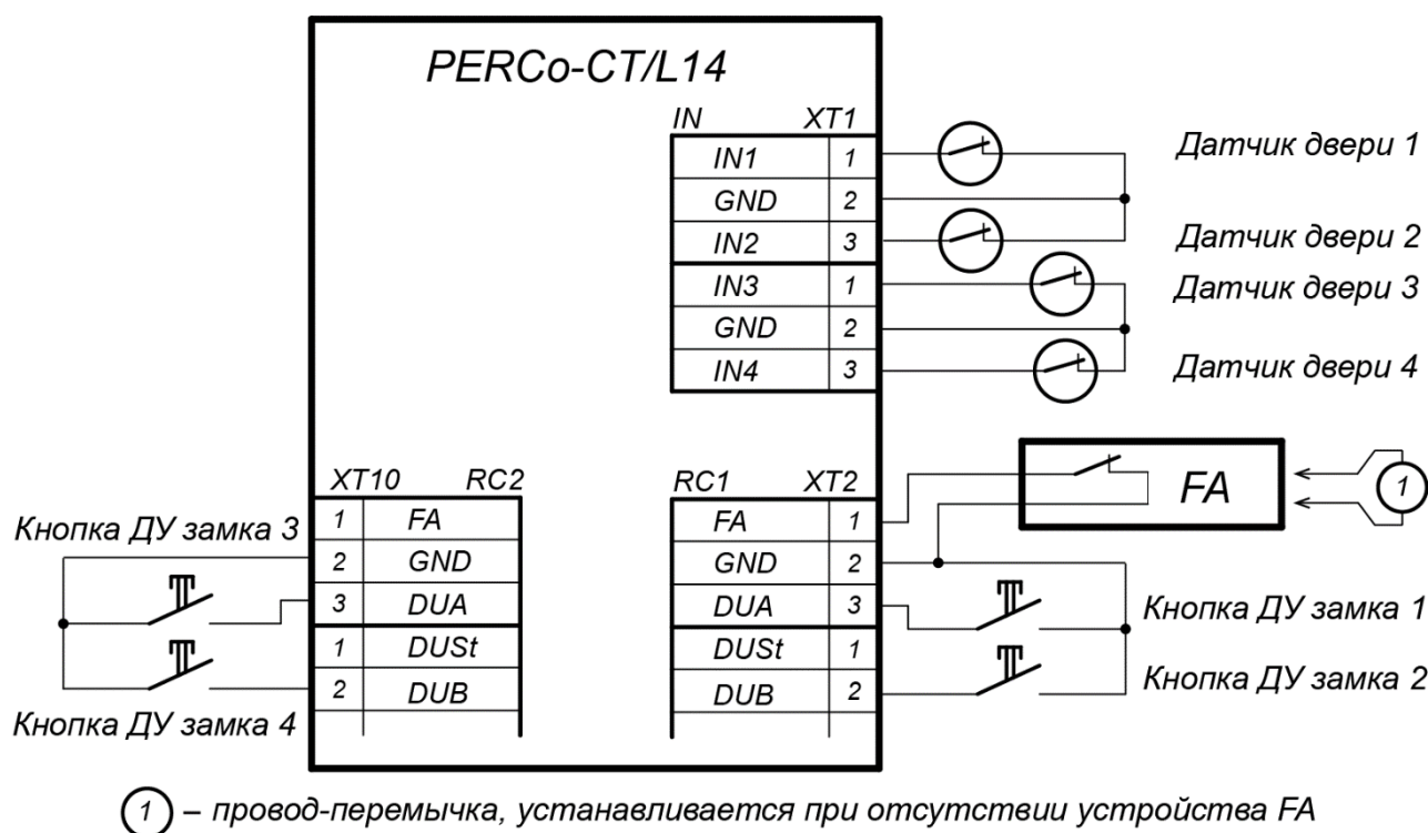
Рисунок 6. Схема подключений кнопок ДУ и датчиков двери
