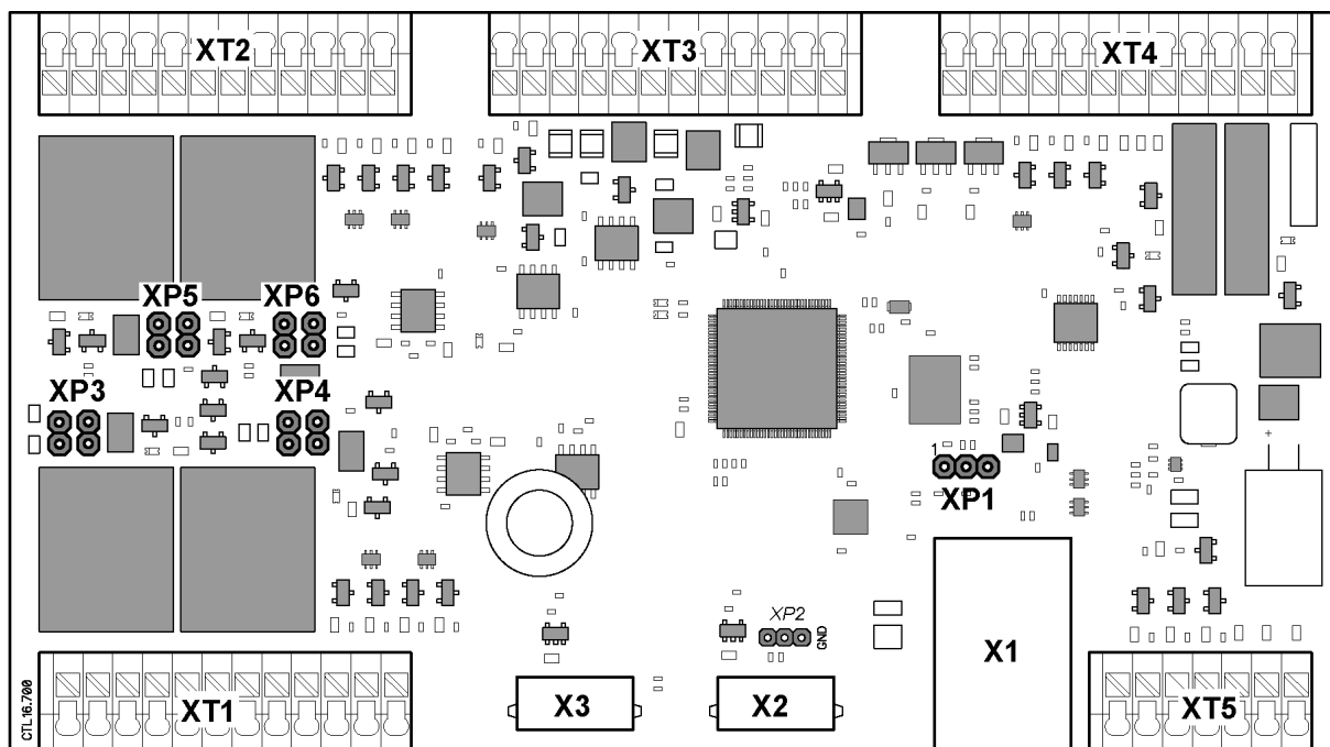
Рисунок 1. Внешний вид платы контроллера
