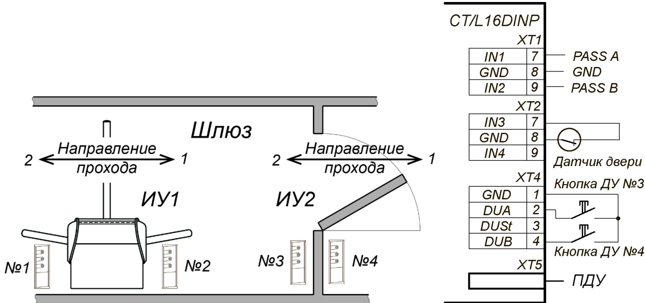
Рисунок 22. Схема шлюза из турникета и замка
