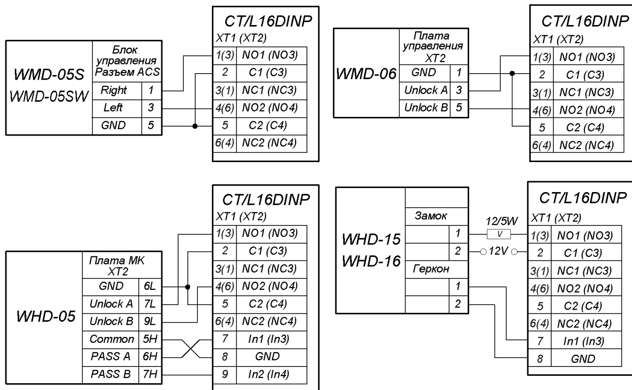
Рисунок 7. Схемы подключений калиток
