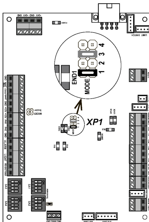
Рисунок 10. Расположение джампера «MODE1» при левостороннем положении стрелы
