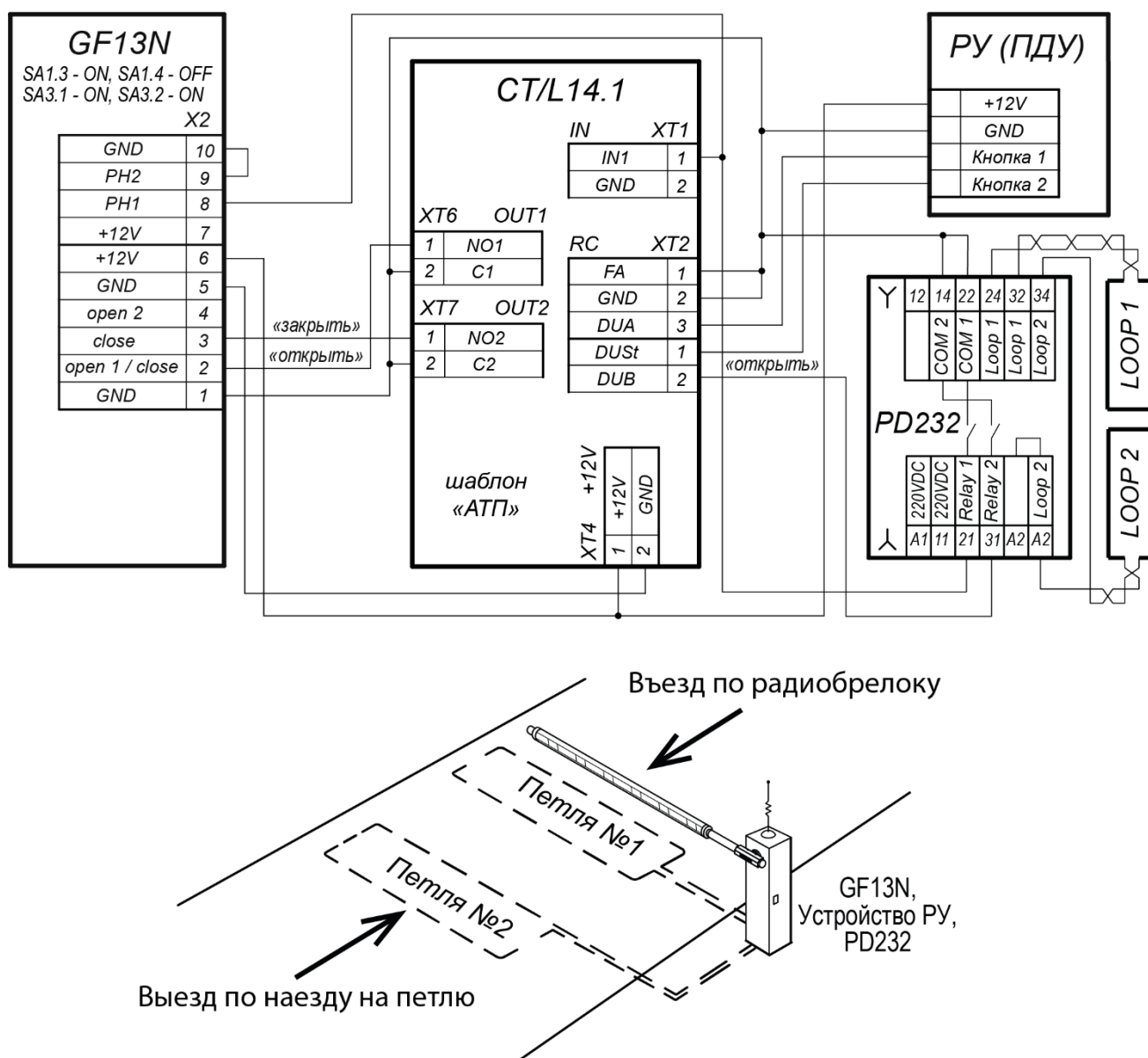
Рисунок 15. Вариант схемы подключения датчика индукционной петли для управления шлагбаумом с двусторонним проездом
