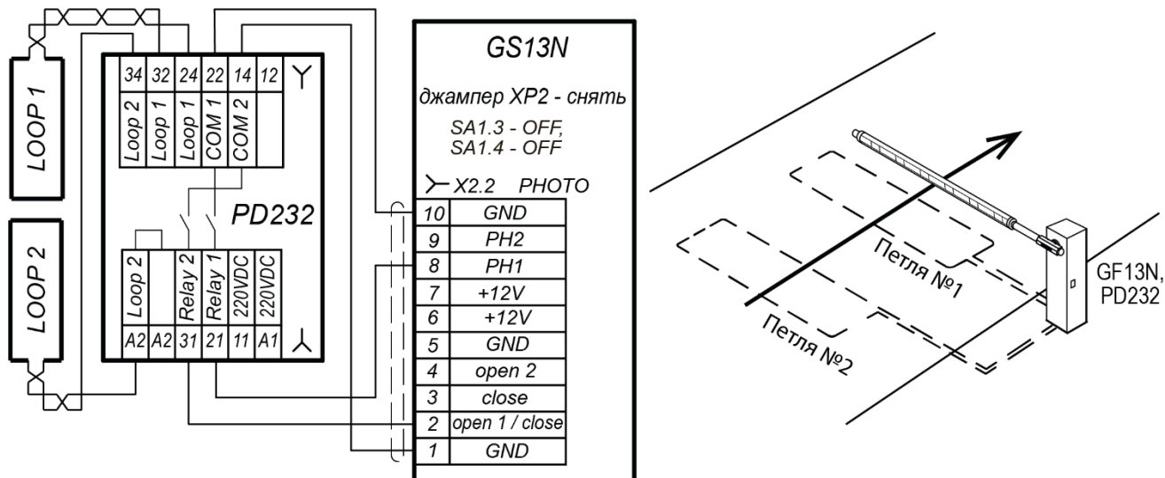
Рисунок 16. Вариант схемы подключения датчика индукционной петли для управления шлагбаумом с односторонним проездом
