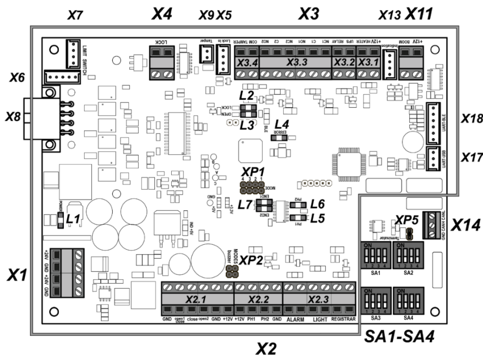
Рисунок 3. Внешний вид платы управления и расположение элементов
