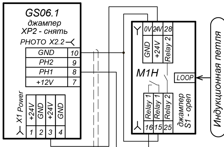
Рисунок 19. Схема подключения одноканального датчика M1H
