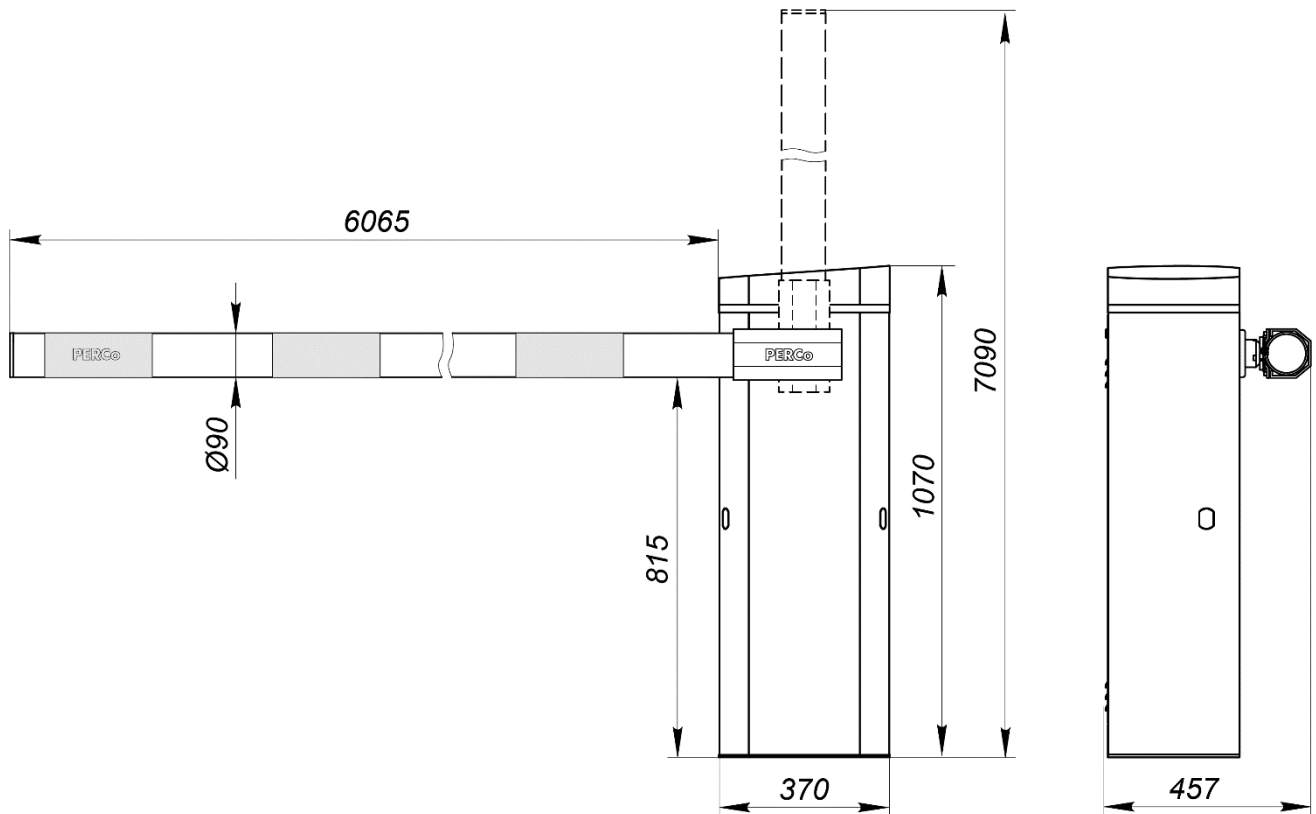
Рисунок 1. Габаритные размеры шлагбаума
