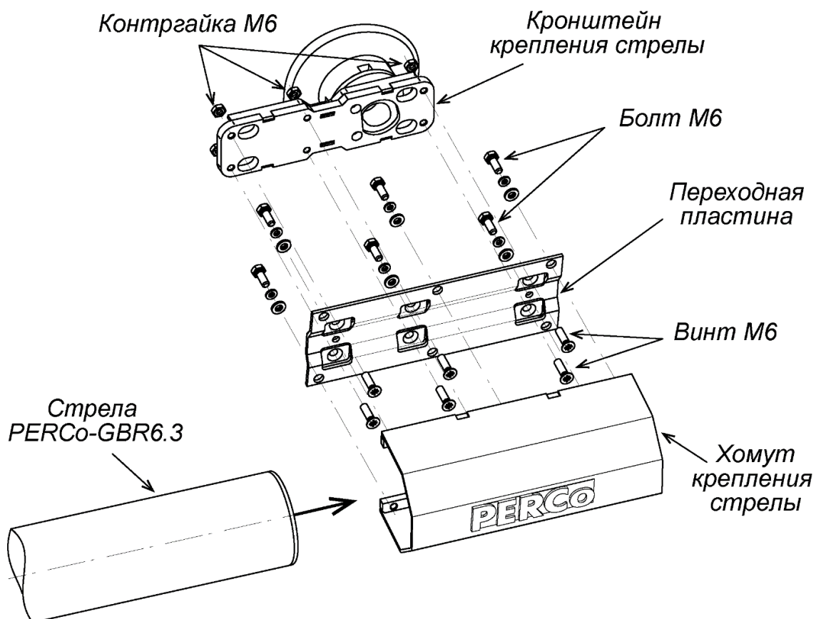
Рисунок 14. Монтаж стрелы PERCo-GBR6.3
