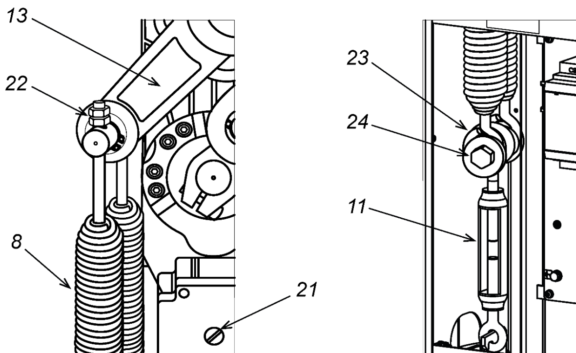
Рисунок 15. Установка балансировочных пружин
