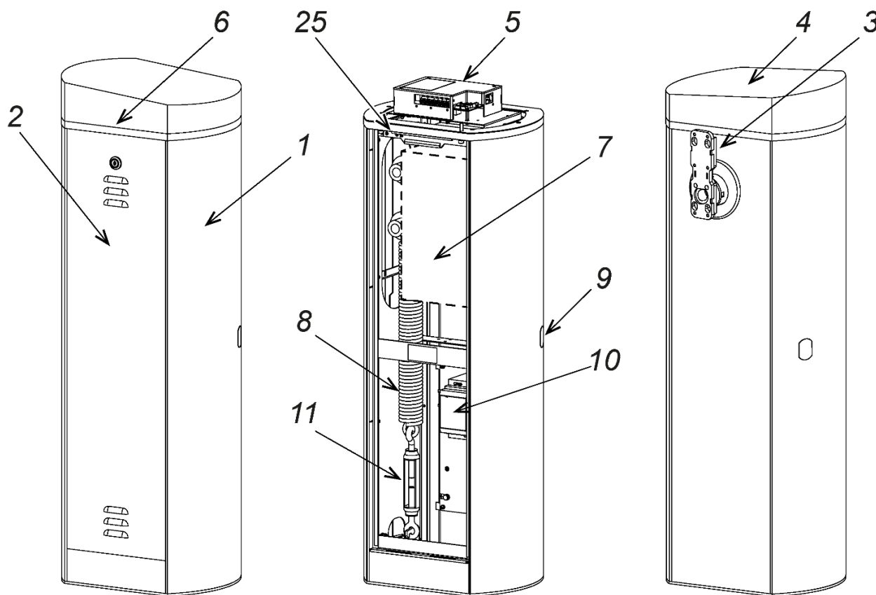
Рисунок 2. Устройство шлагбаума
