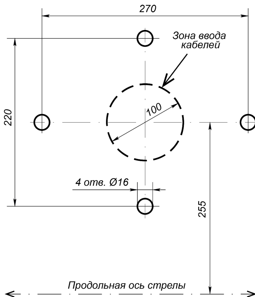
Рисунок 7. Разметка установочных отверстий шламбаума
