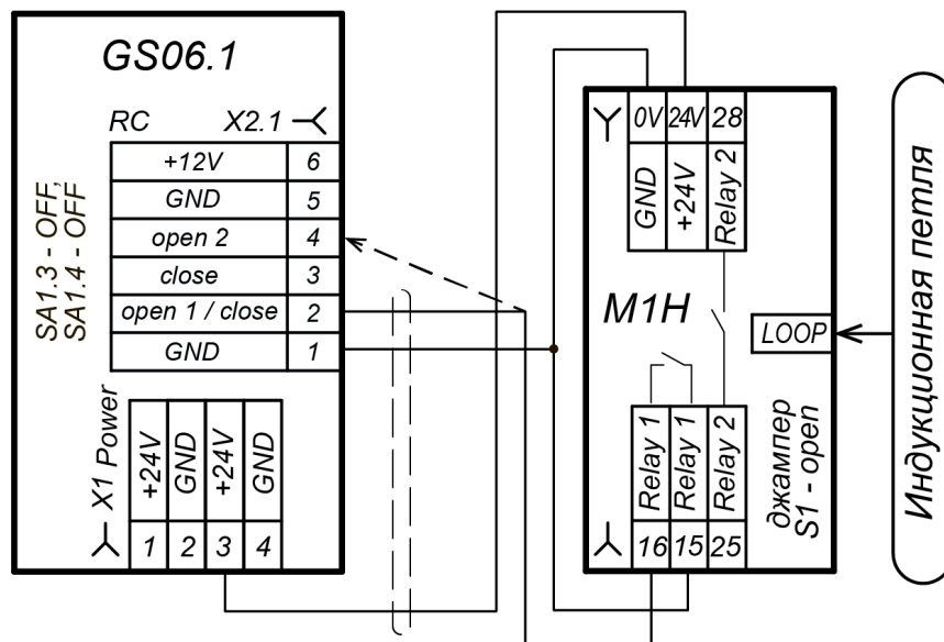
Рисунок 21. Вариант схемы подключения датчика индукционной петли для управления шлагбаумом с односторонним проездом
