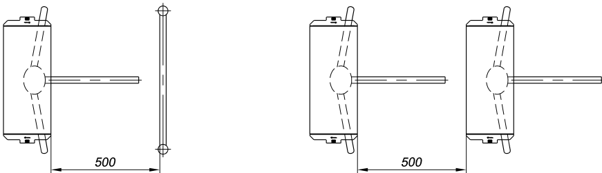
Рисунок 5 — Рекомендации по организации зоны прохода
