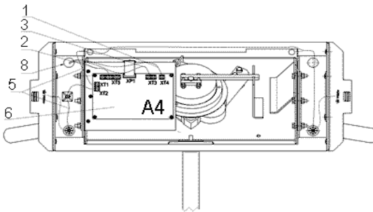
Рисунок 7 — Схема прокладки кабелей в стойке ЭП
