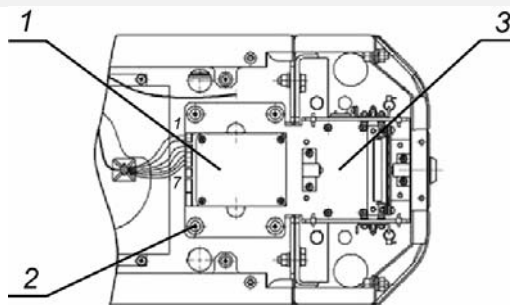
Рисунок 14. Механизм картоприемника
