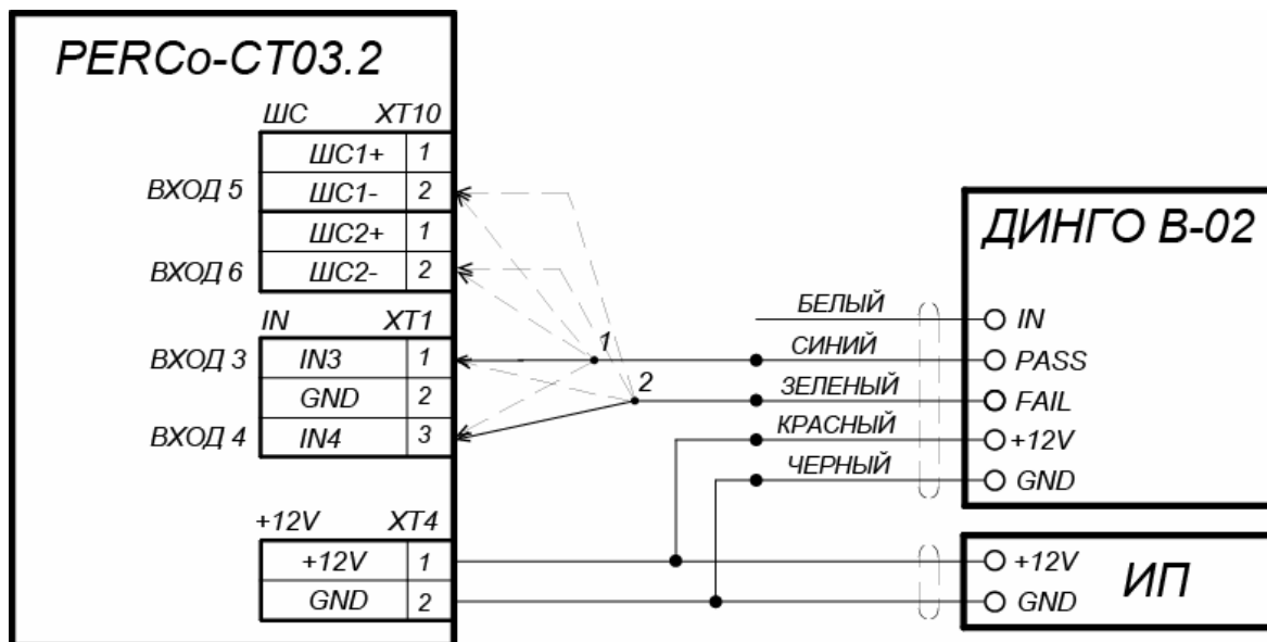
Рисунок 16. Схема подключения алкотестера «Алкобарьер» (ООО «Алкотектор»)
