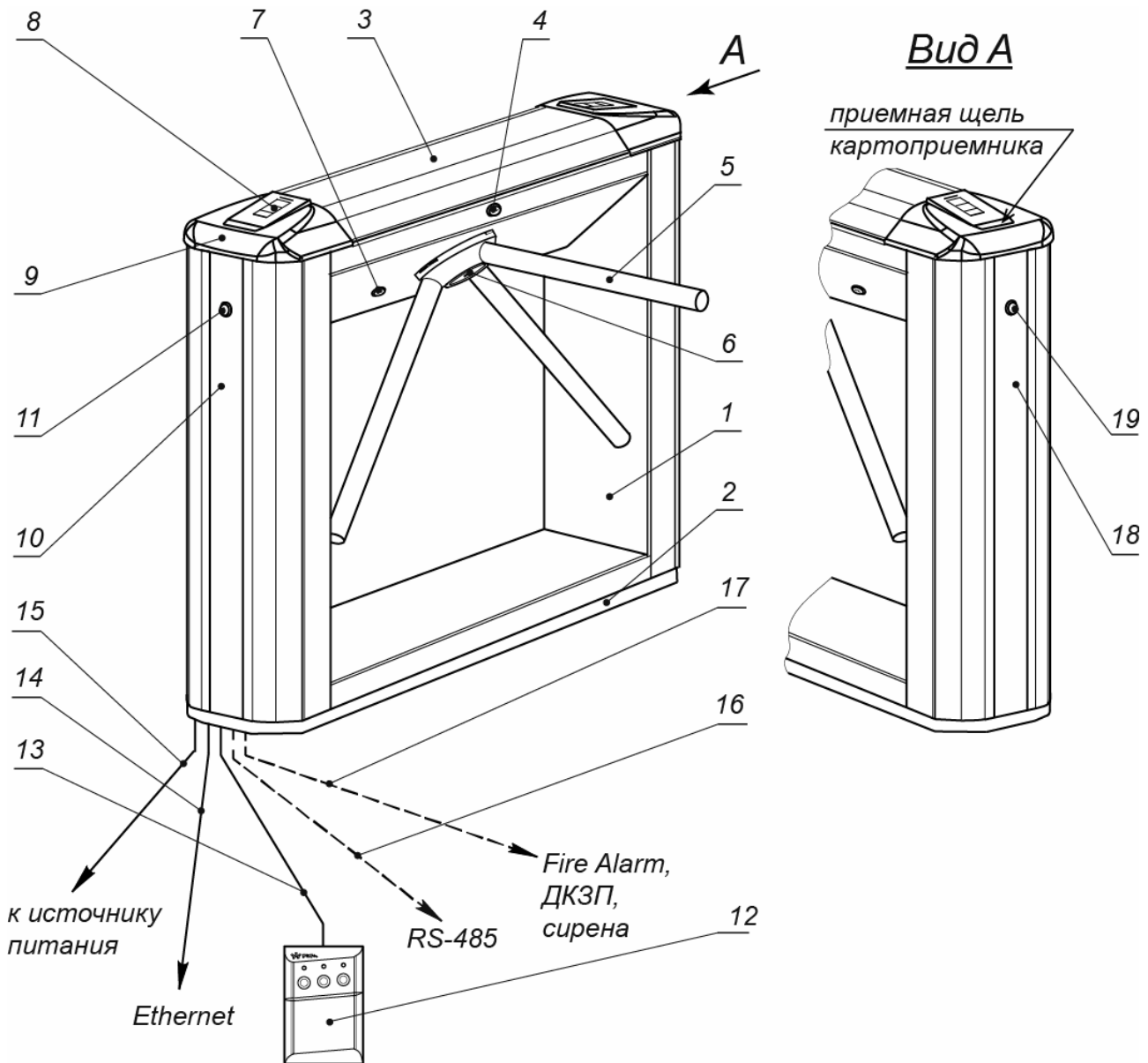
Рисунок 1. Устройство ЭП
