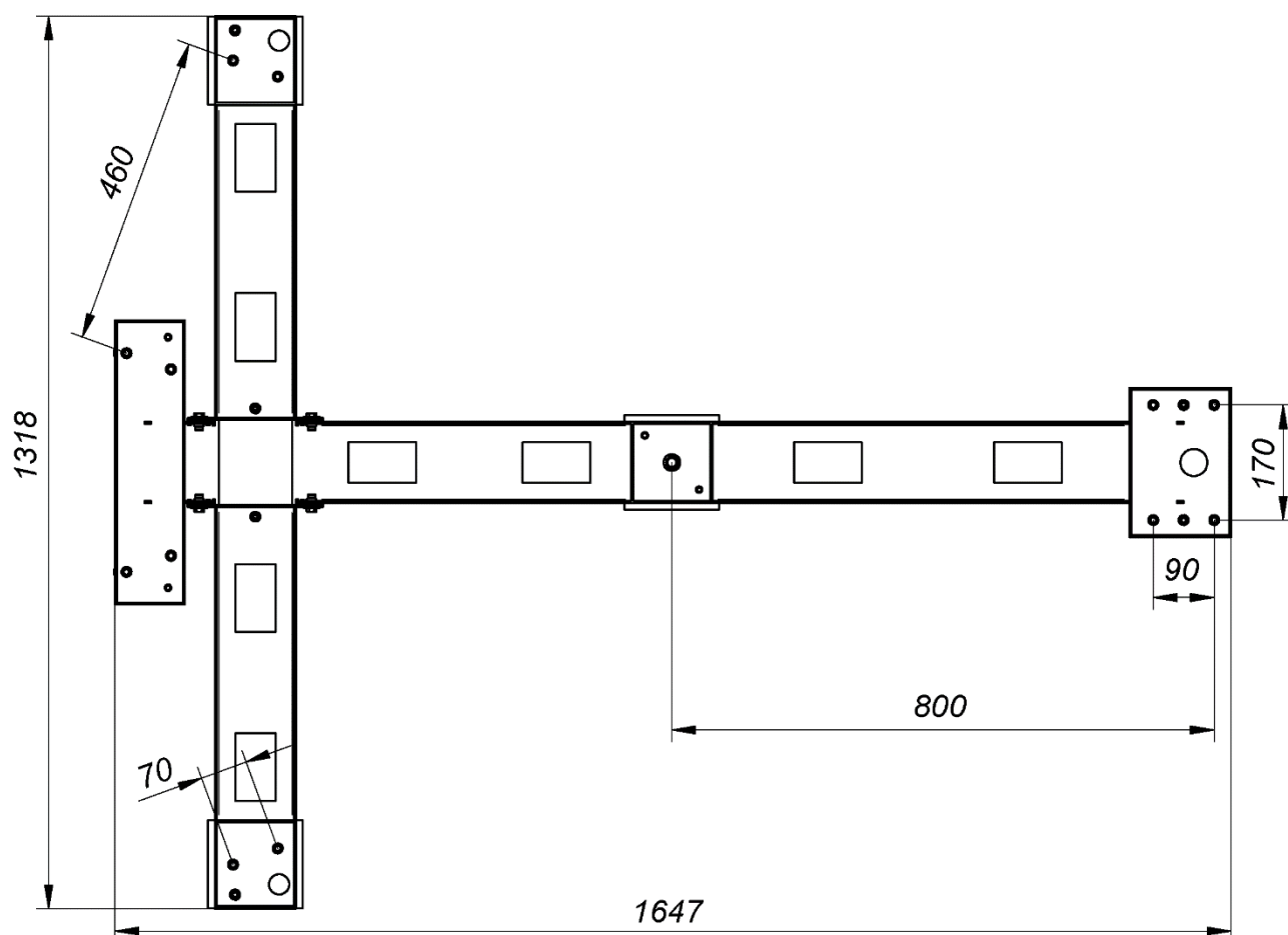
Рисунок 1. Габаритные и установочные размеры рамы
