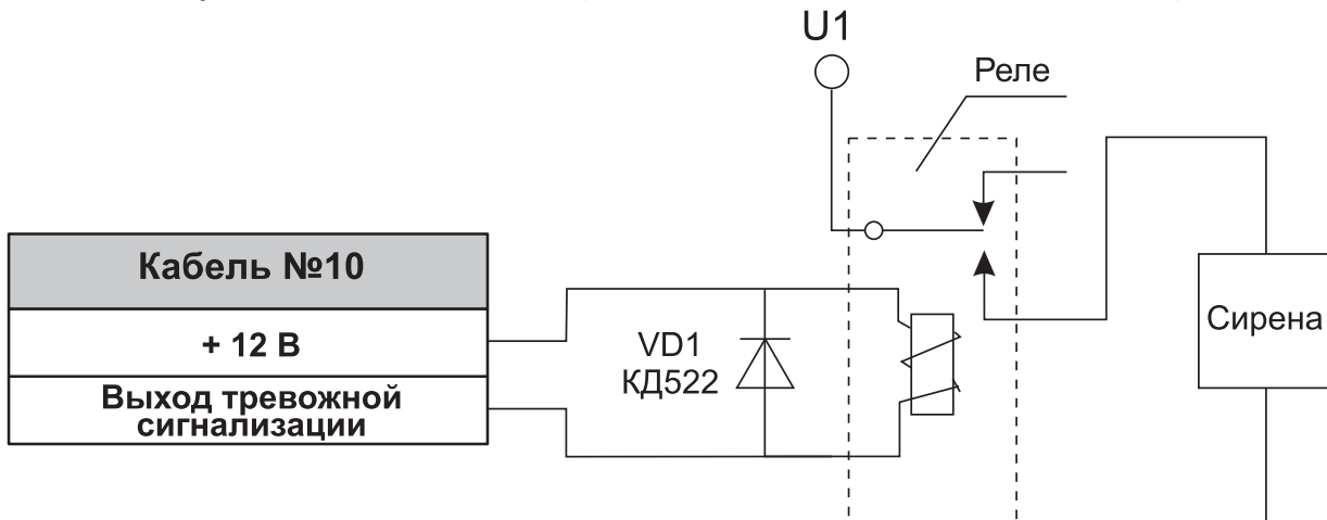
Рисунок 3 - Пример гальванической развязки цепи
