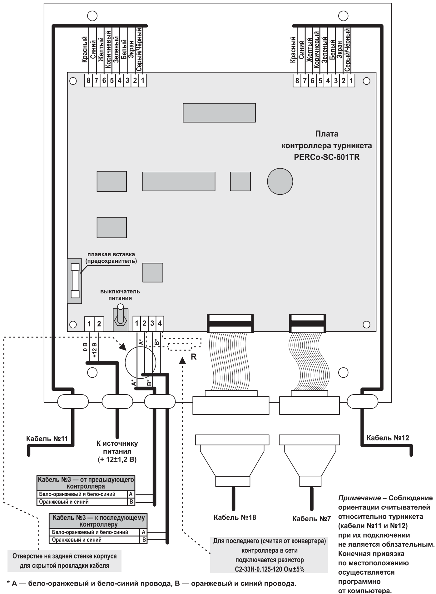
Схема 10- Схема монтажа контроллера роторного турникета PERCo-SC-601TR
