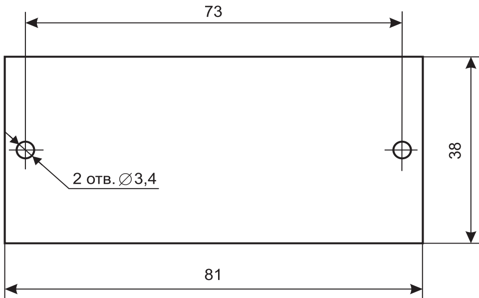
Рисунок 2 - Разметка отверстий для установки пульта руководителя PERCo-H-600
