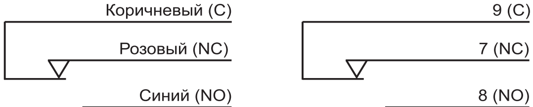
Рисунок 4 - Выходное реле замковых контроллеров PERCo-SC600LH (LE) с указанием цвета проводов. Выходное реле замковых контроллеров PERCo-SC601LH (LE) с указанием номеров контактов
