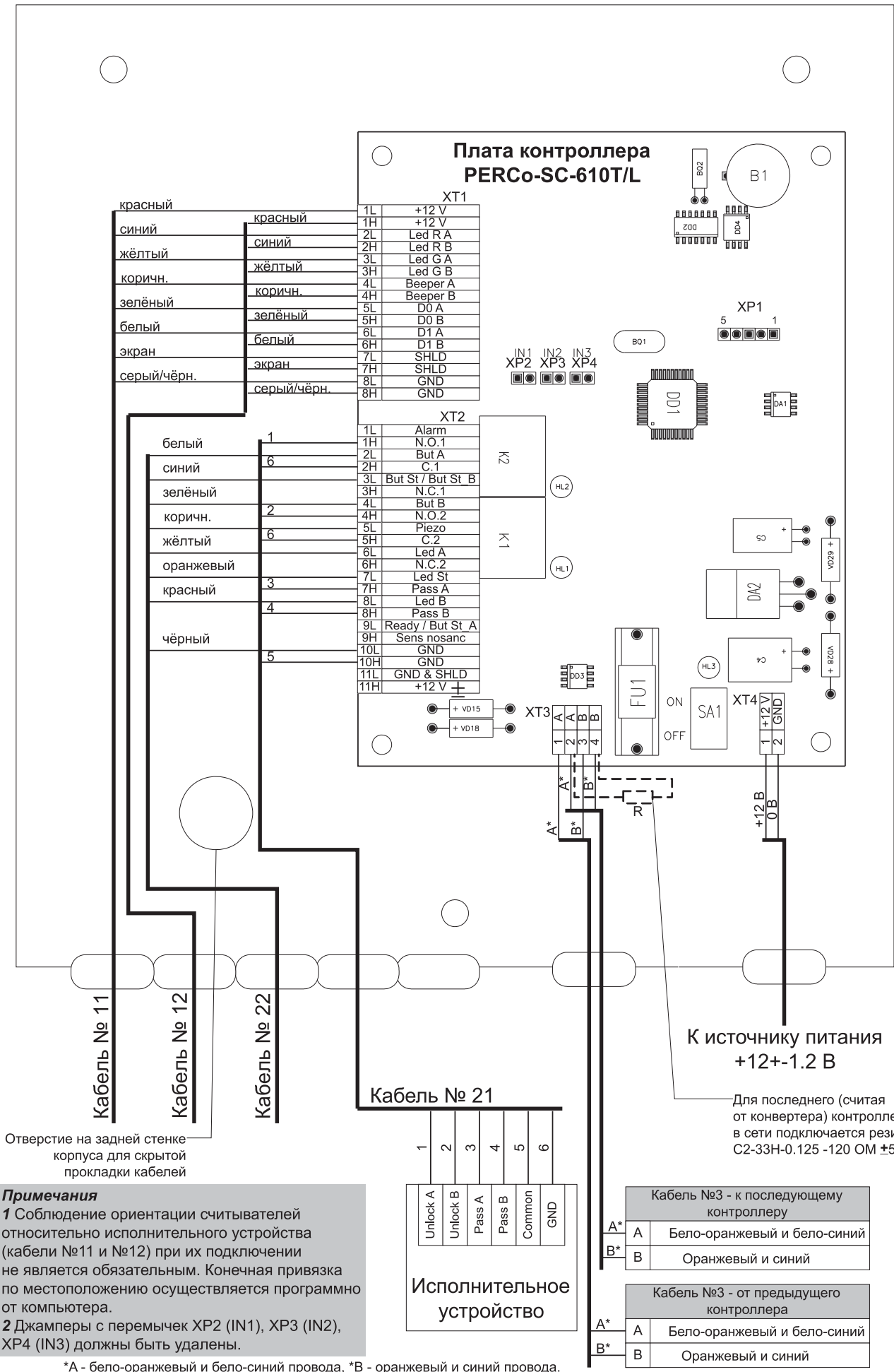
Схема 13- Схема монтажа контроллера PERCo-SC-610T/L (вариант "Турникет")
