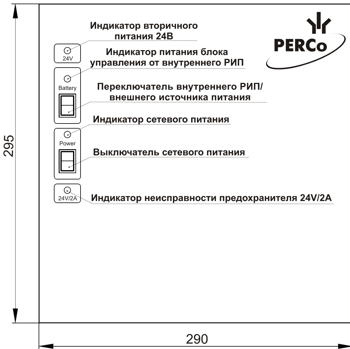
Рисунок 3 - Блок управления
