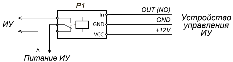
Схема гальванической развязки управления исполнительным устройством
