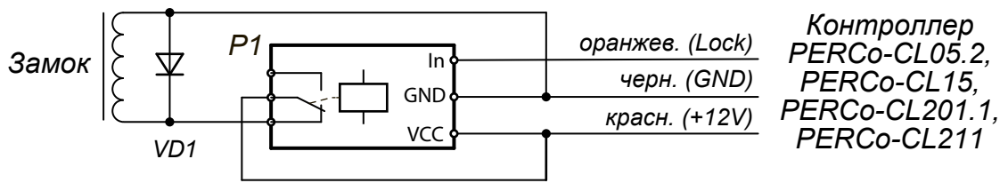
Схема подключения нормально открытого замка к контроллерам PERCo-CL05.2, PERCo-CL15, PERCo-CL15.3, PERCo-CL15.7, PERCo-CL201.1, PERCo-CL211.3, PERCo-CL211.9
