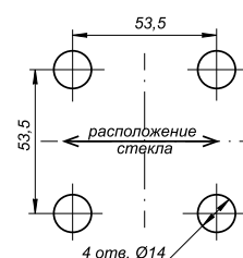
Разметка отверстий для мини-стойки
