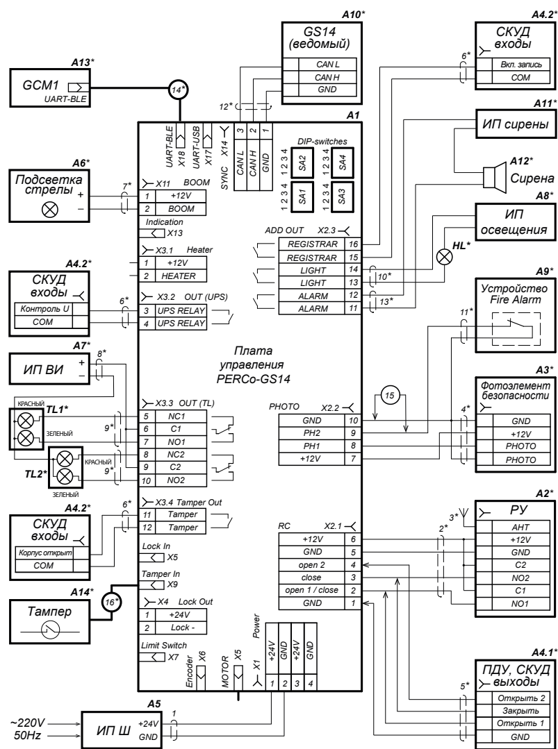
Схема электрических соединений шлаббаума GS14
