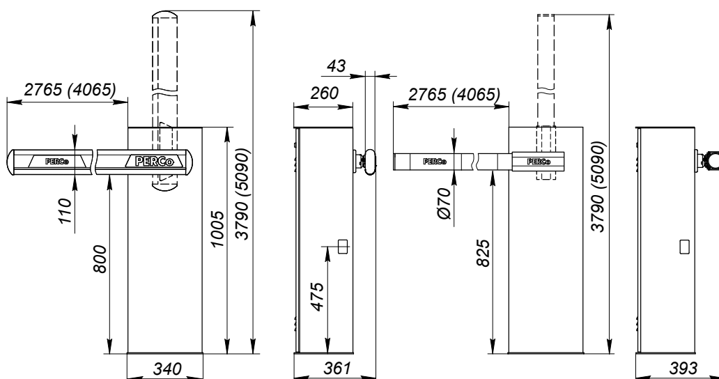
Габаритные размеры
